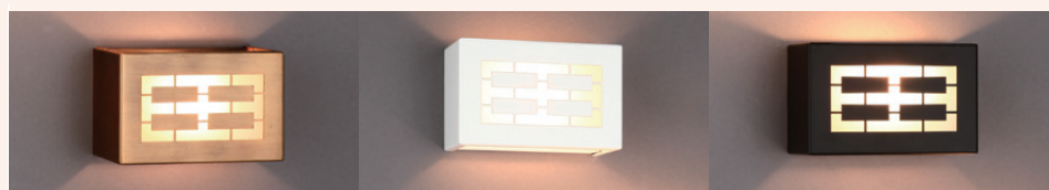
▶LD 데코 B/R (황금브론즈, 백색, 흑색) ▶Size : W160×D80×H100 ▶Lamp : E17 ※LED 램프 전용
